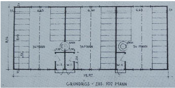
Abb.: Grundriss einer Baracke aus Bauakte Brötzingen Talweg 10 (Stadtarchiv Pforzheim)
